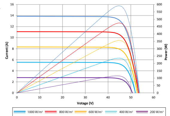
电流-电压 & 功率-电压曲线图 (590S)
